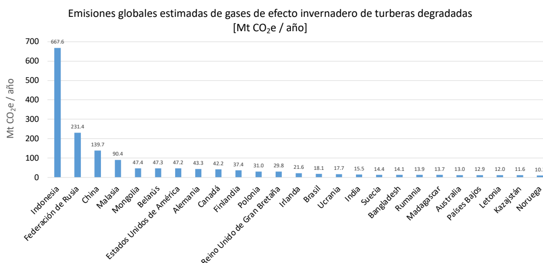
Figura 0.3: Emisiones globales estimadas de gases de efecto invernadero de turberas degradadas de los 25 principales países emisores. Los cálculos se basan en el área drenada de turberas para la silvicultura, la agricultura y la extracción de turba y los factores de emisión del IPCC (2014), incluidos CO 2 , CH 4 , N 2 O, DOC y emisiones de zanjas. Incluye solo las emisiones netas de GEI en el sitio. No están incluidas las emisiones de incendios forestales.
