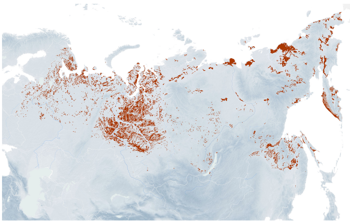
Distribución de turberas en la Federación de Rusia ■ turbera (profundidad \geq 30 cm)
