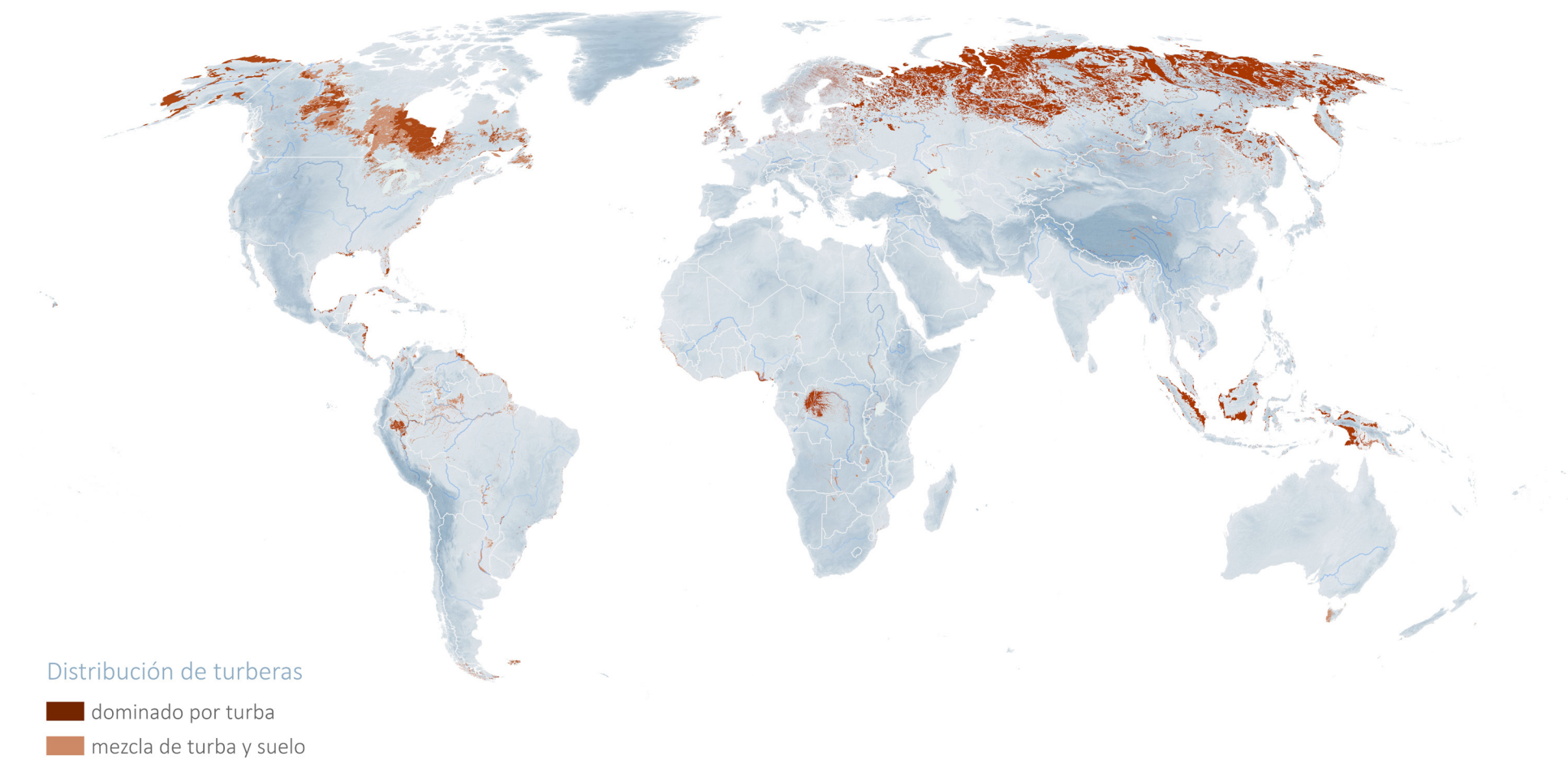
Figura 0.2: Mapa Mundial de Turberas 2.0.
